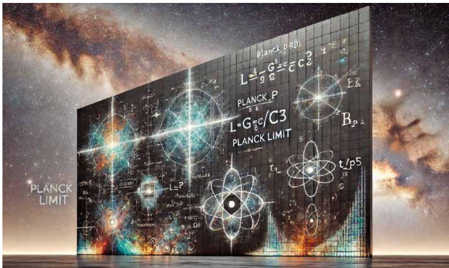
Le Mur de Planck est un concept fascinant en physique théorique qui nous plonge dans les premiers instants de l'Univers.
